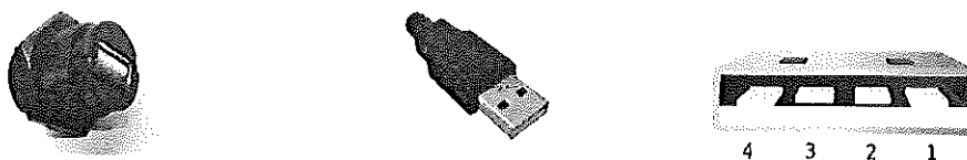
(a) 電源供應器端 (b) 通訊模組端 (c) 通訊模組端腳位順序
