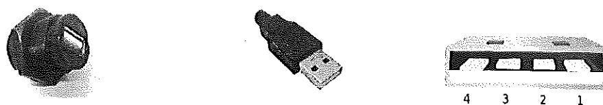
(a) 電源供應器端 (b) 通訊模組端 (c) 通訊模組端腳位順序
