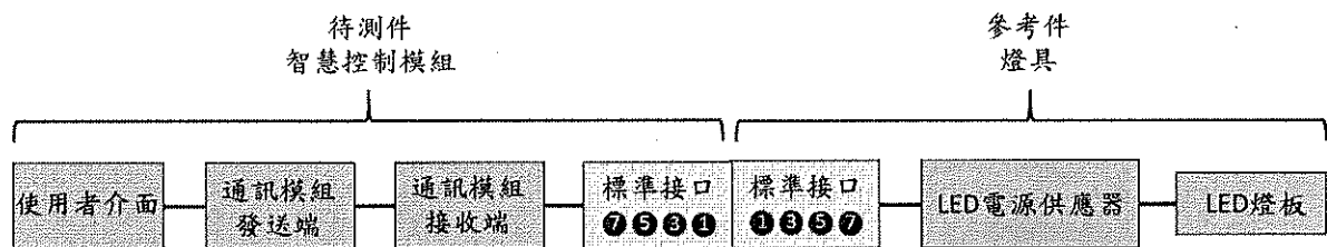
圖6 待測件智慧控制模組對接 ITRI 參考件燈具之測試架構
