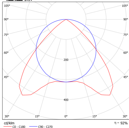
極座標
